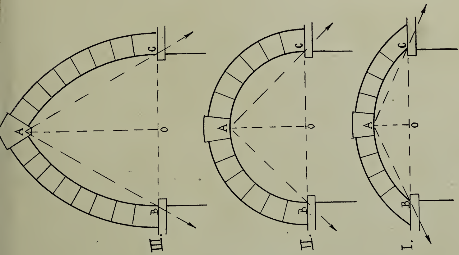
FIGURA 101—Empuje de los arcos según la altura de su flecha: I, arco rebajado; II, arco de medio punto; III, arco apuntado.
